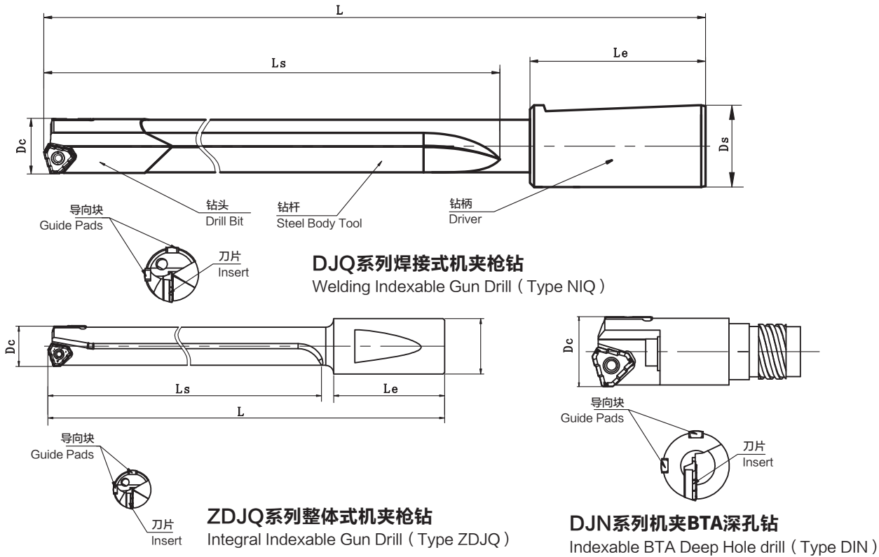
N/ZN型机夹式深孔钻通用配置表 Products List For Indexable Deep Hole Drill(Type D/ZD)
