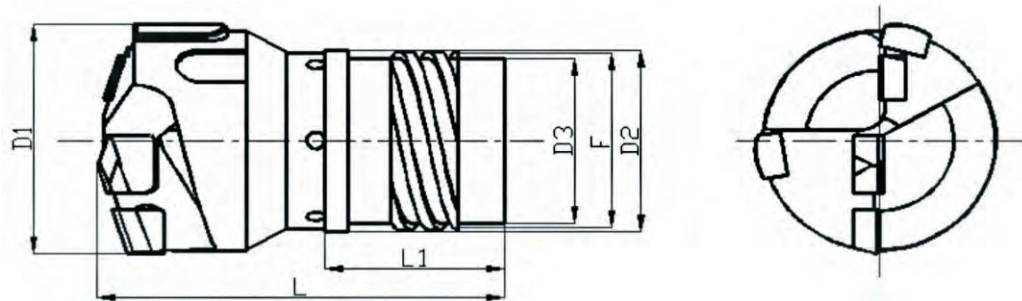
P型钻头系列表
